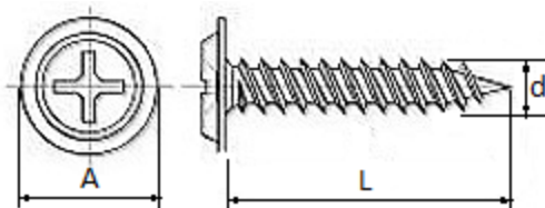
Винт с широка периферия, самонарезен, поцинкован, PH
