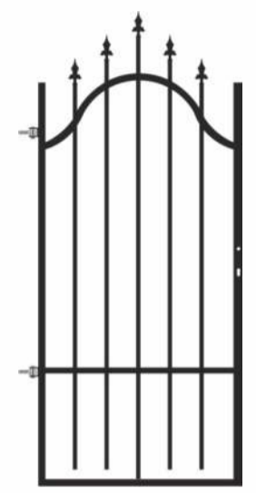
ВРАТА ОГРАДНА ЛЯВА/ДЯСНА 0,90 m x 1,70-2,00 m
