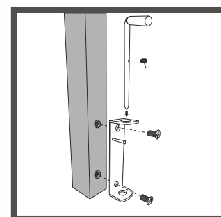
СЮРМЕ ЗА ДВУКРИЛА ВРАТА ДОЛНО
