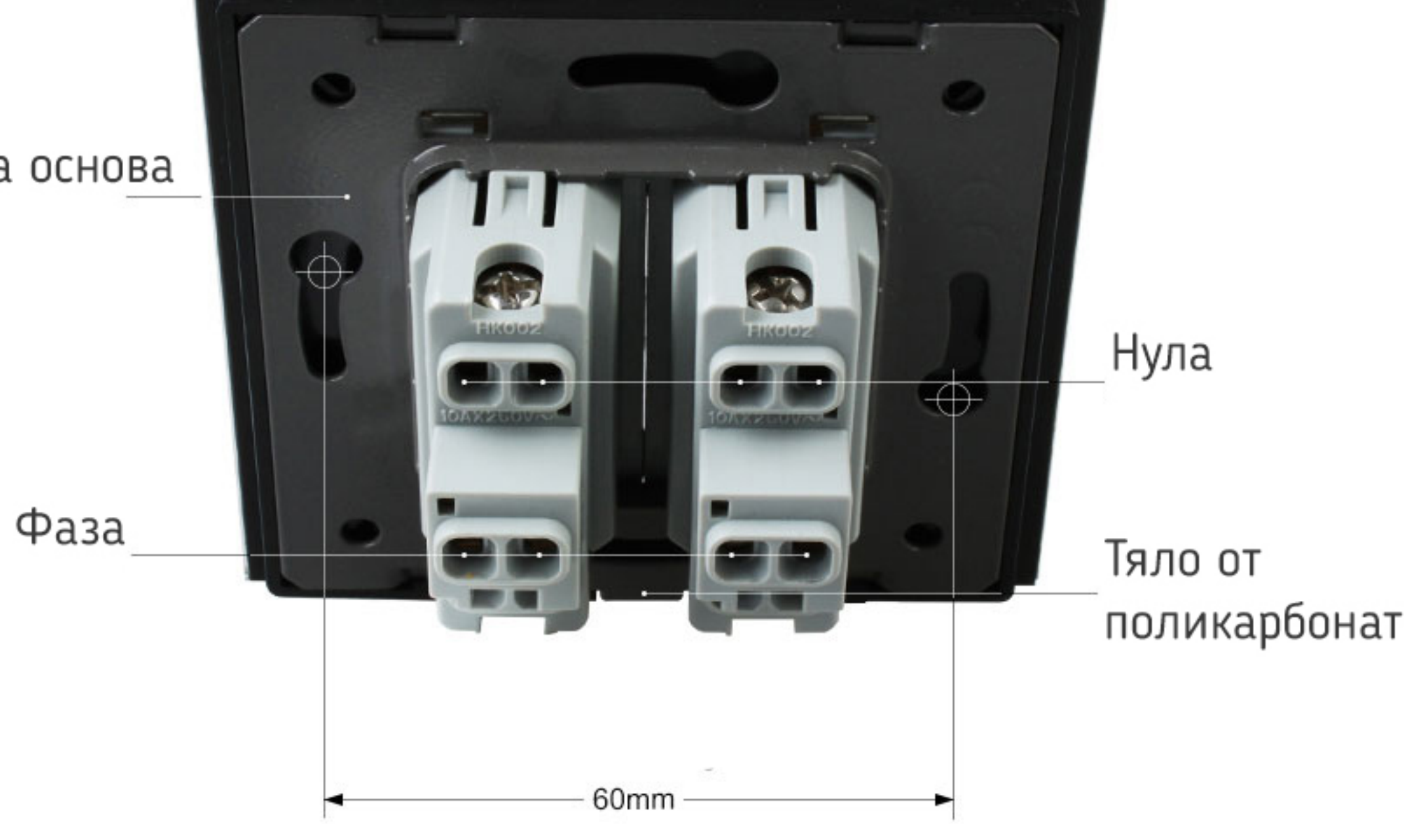
Съклен панел
